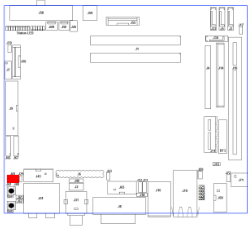
ETXexpress® miniBaseboard
